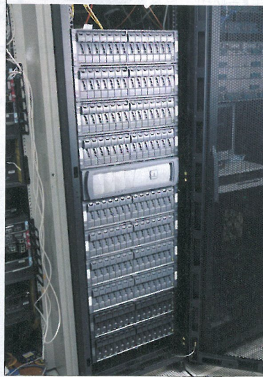
教院採用的 NetApp 儲存方案，主要包括一對 FAS3240 儲存陣列，以及 NetApp MetroCluster 方案。
